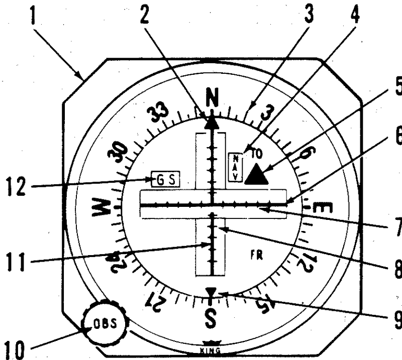
INDICATEUR VOR/ILS KI 204/206 (TYPE)
