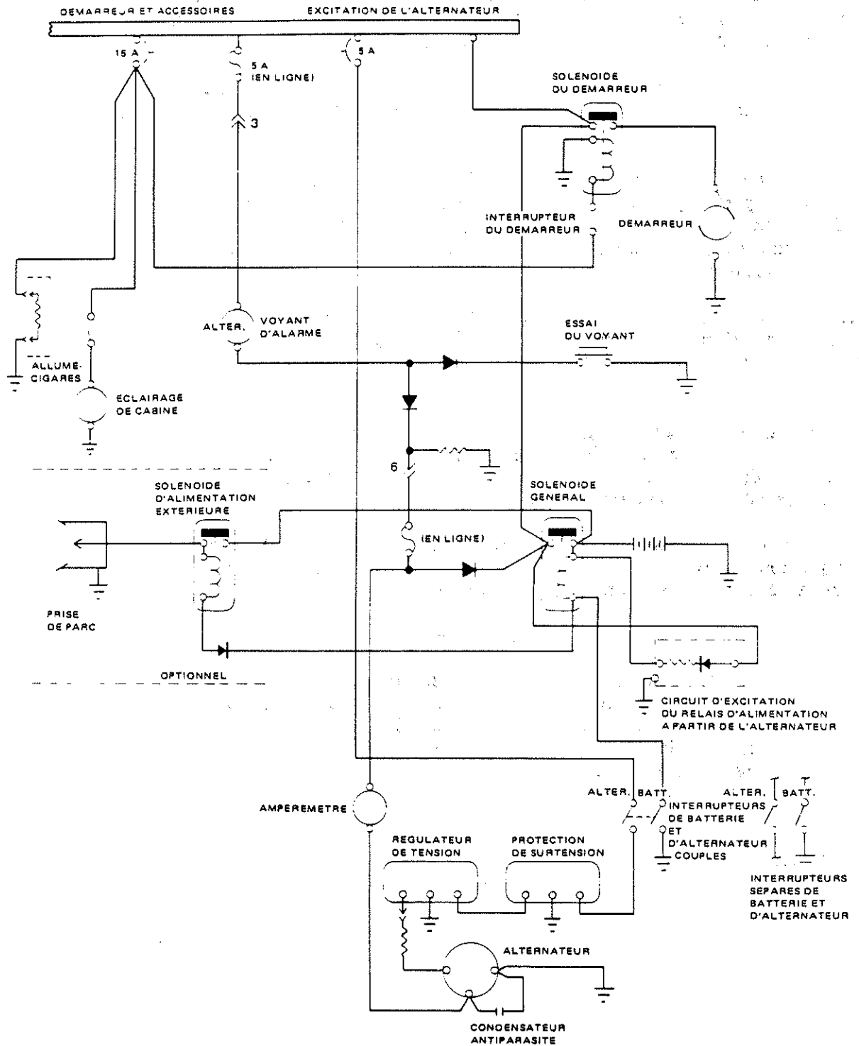
SHEMA DE PRINCIPE DE L'ALTERNATEUR ET DU DEMARREUR
