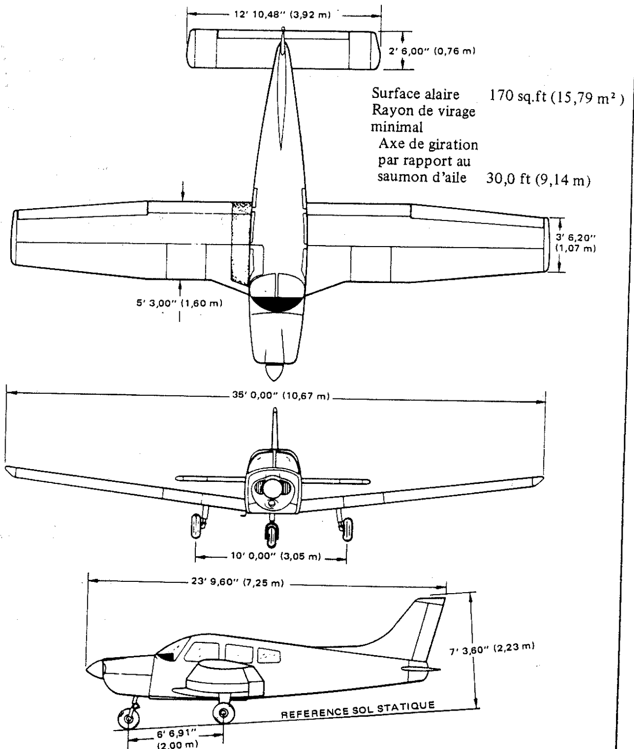
PLAN TROIS VUES
