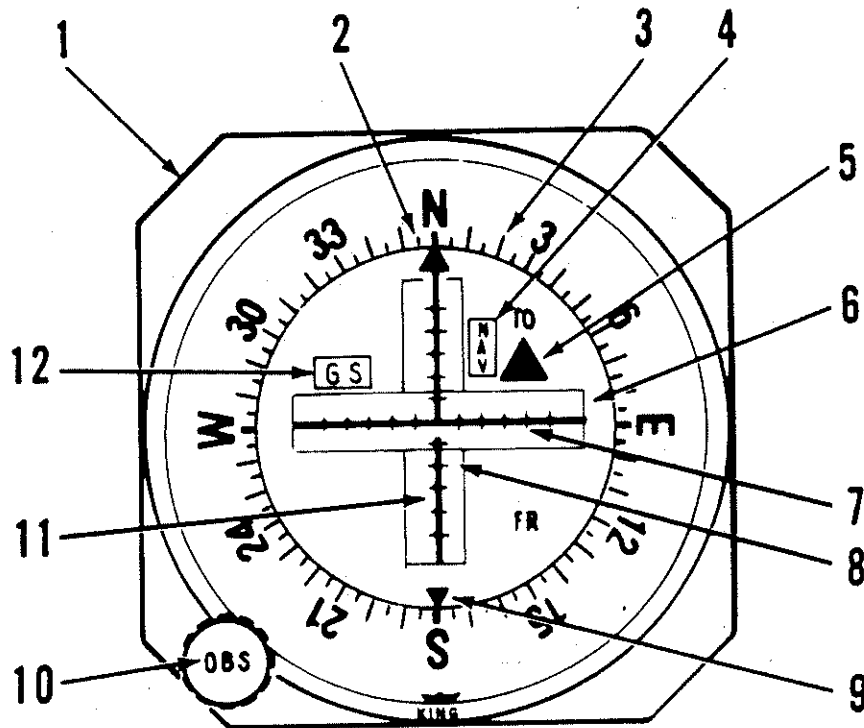
INDICATEUR VOR/ILS KI 204/206 (TYPE)
